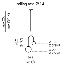
DECOR_1 pendant
