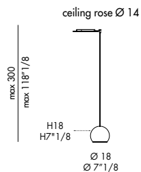
CHERRY_1 pendant
