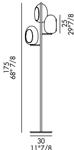
FOS_floor
