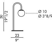
DECOR_1 table
